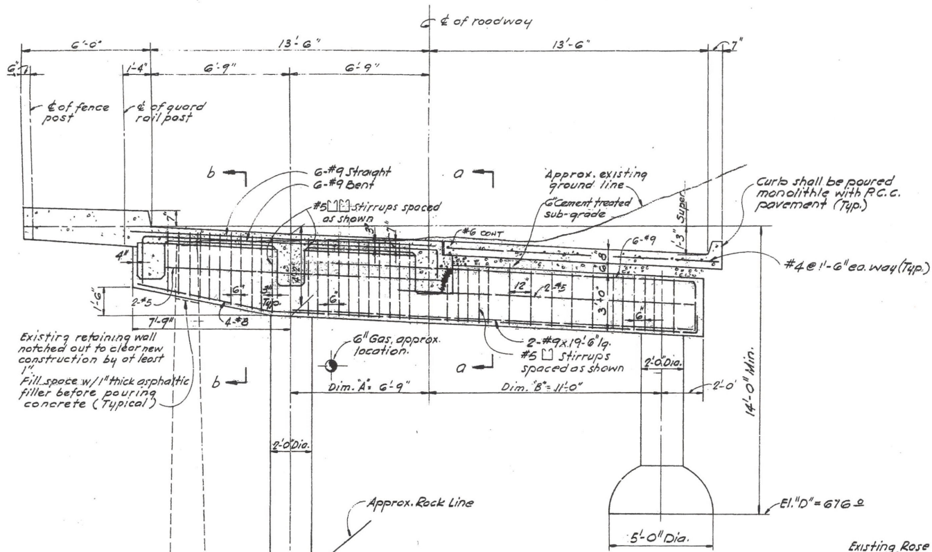
PILE BENT #2 AT STA. 7+85.25 Scale: 3/8" = 1'-0"
