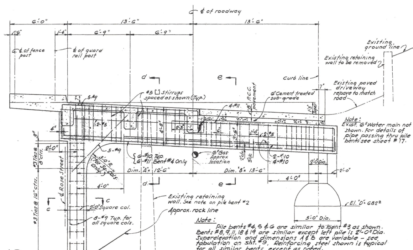
PILE BENT #3 AT STA. 8+09.25 Scale: 3/8" = 1'-0"
